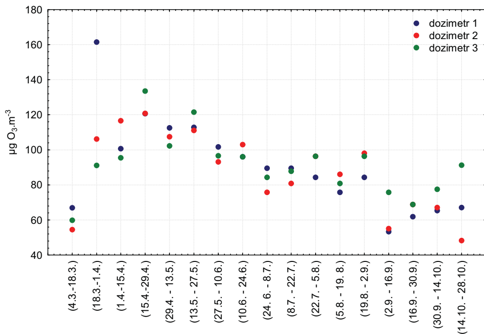
Obr. 4.2.9.6: Vývoj koncentrací ozonu Development of ozone concentrations
