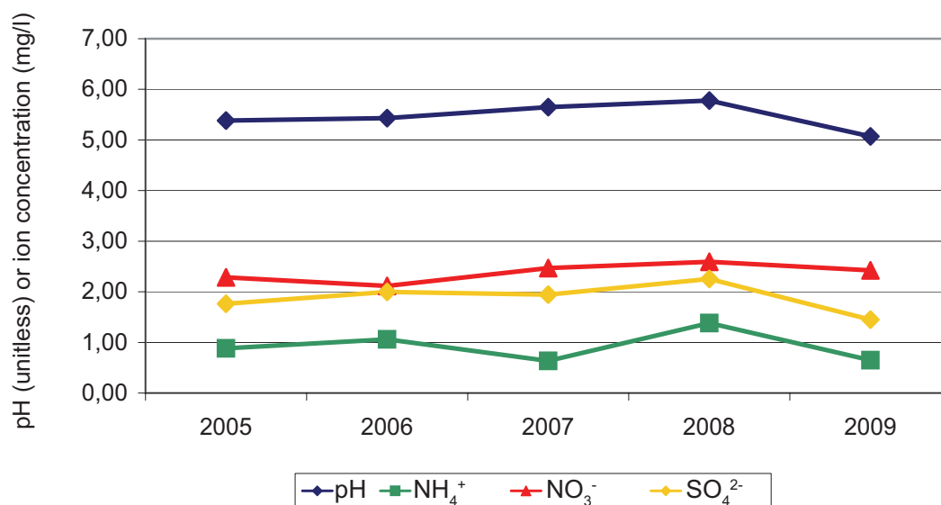
Obr. 4.2.7.6: Vývoj pH a průměrné koncentrace iontů – volná plocha 2005 – 2009 Mean ion concentration and pH – bulk 2005 – 2009
