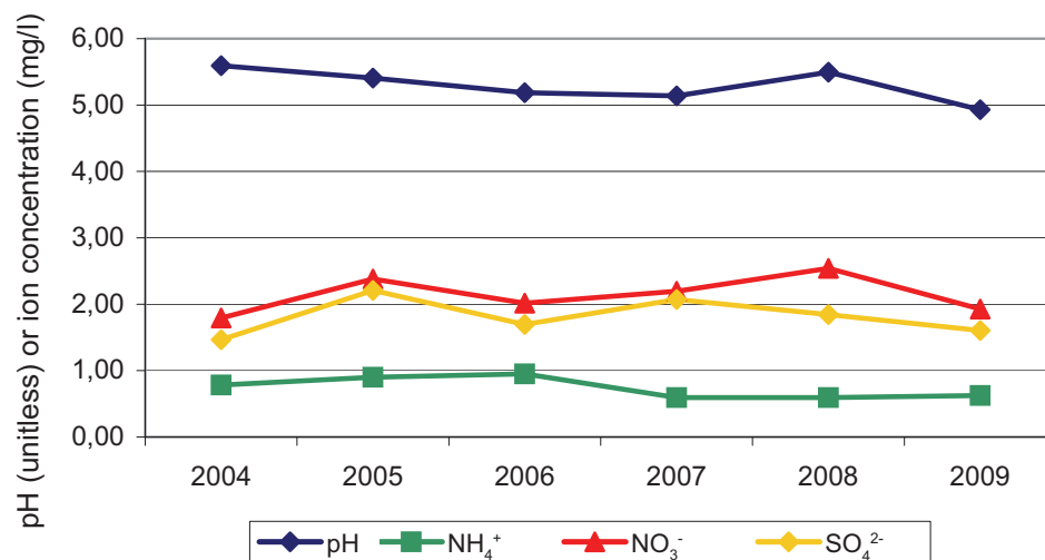
Obr. 4.2.5.6: Vývoj pH a průměrné koncentrace iontů – volná plocha 2004 – 2009 Mean ion concentration and pH – bulk 2004 – 2009
