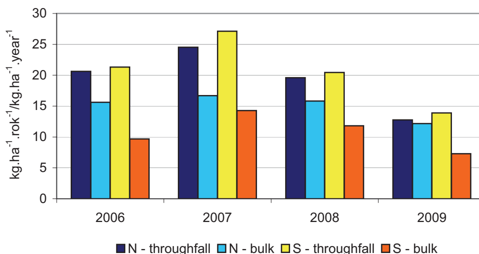
Obr. 4.2.9.3: Celková depozice dusíku a síry ( \text{kg}\cdot\text{ha}^{-1}\cdot\text{rok}^{-1} ) Total nitrogen and sulphur deposition ( \text{kg}\cdot\text{ha}^{-1}\cdot\text{year}^{-1} )
