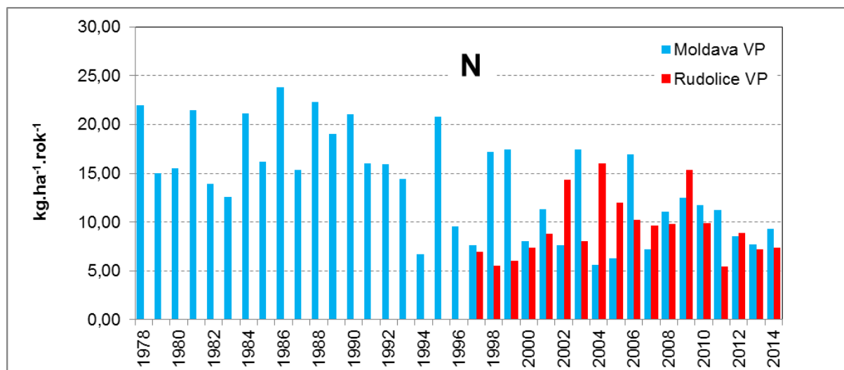
Obr. 1.10: Vývoj depozice dusíku na volné ploše na stanicích Moldava a Rudolice v Horách (podle dat VÚLHM a ČHMÚ)
