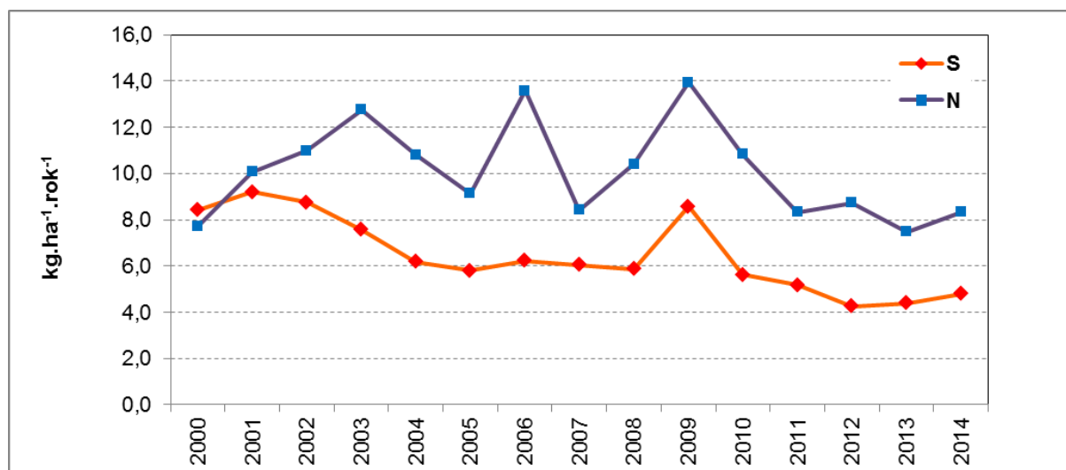
Obr. 1.11: Vývoj depozice síry a dusíku na volné ploše (průměrné hodnoty ze stanic Moldava a Rudolice v Horách) v letech 2000-2014 (podle dat VÚLHM a ČHMÚ)
