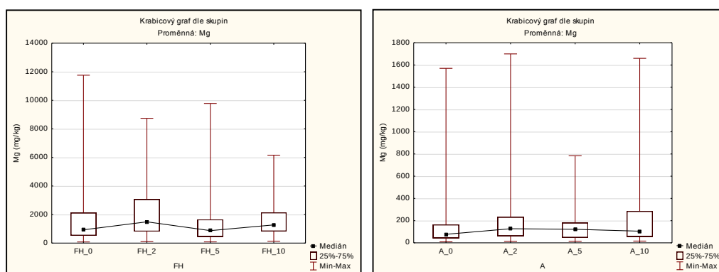
Obr. 2.13: Vývoj přístupného hořčíku v období dvou, pěti a deseti let po vápnění v humusové vrstvě (FH) a v humusem ovlivněném minerálním horizontu (A)
