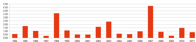
Obr. 6: Vývoj indexu mortality smrku na modelovém území Vojenských lesů a statků ČR, s.p., divize Horní Planá v letech 1994–2011 (příkladová studie, rozloha lesů 16 569 ha) (Jakuš et al. in prep.)
