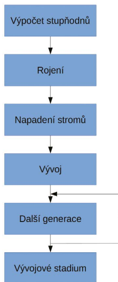
Obr. 21: Modelování vývoje lýkožrouta smrkového
