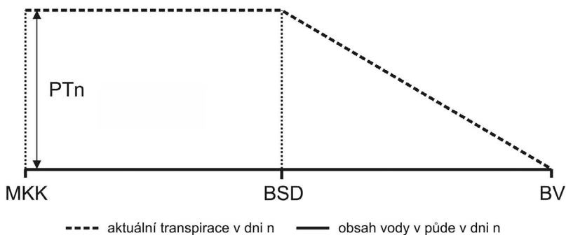
Obr. 13: Schéma vztahu pro stanovení hodnoty aktuální transpirace (přerušovaná čára) na základě aktuálního obsahu vody v půdě (os x). MKK = maximální kapilární kapacita, BSD = bod snížené dostupnosti, BV = bod vadnutí, PT_n = potenciální transpirace v den n
