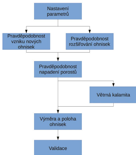
Obr. 20: Výpočet prognózy šíření ohnisek lykožrouta smrkového
