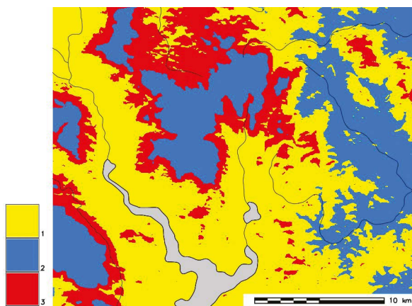
Obr. 10: Prognóza stupně vývoje lýkožrouta smrkového (185. den)
