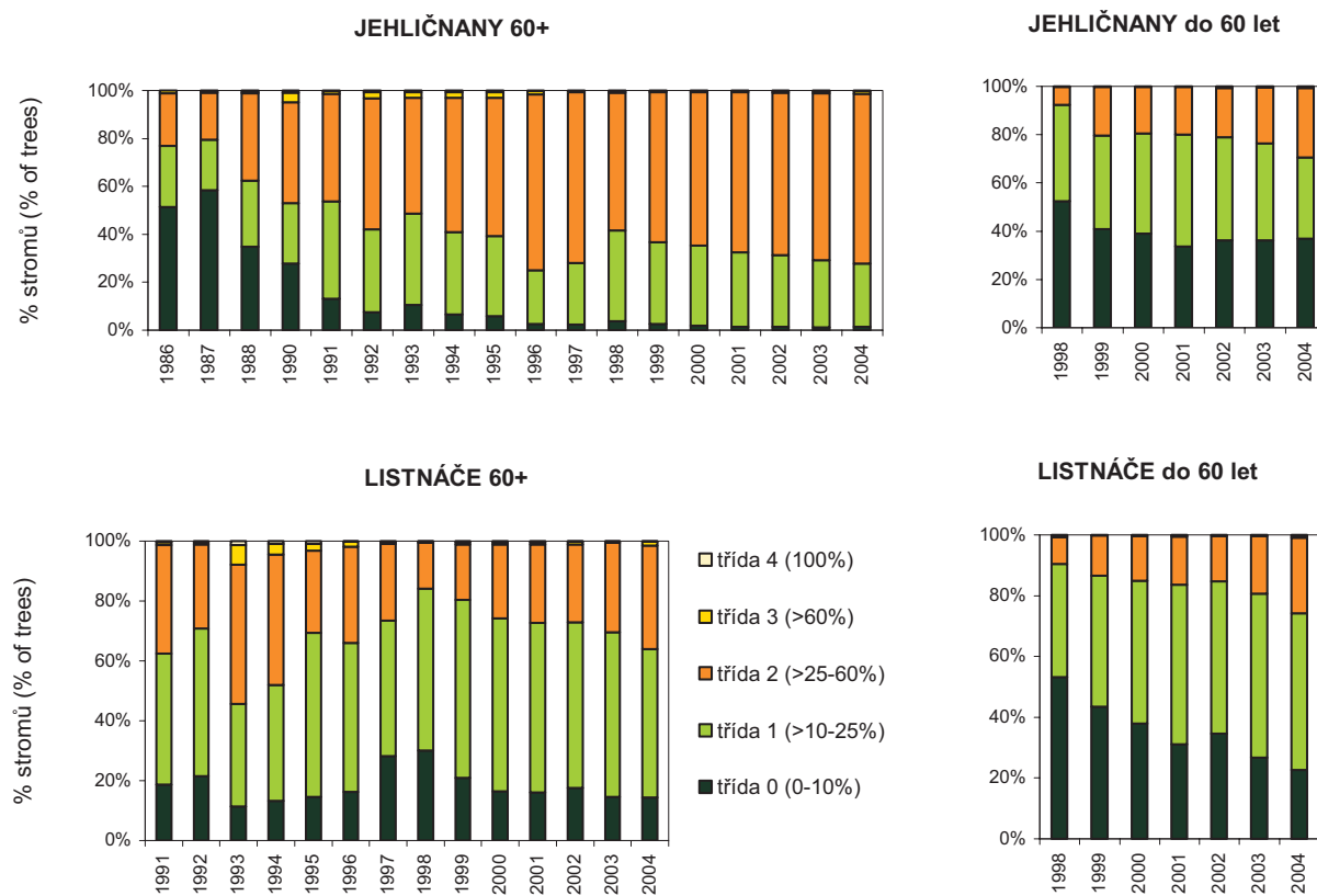
Obr. 48: Zastoupení tříd defoliace u jehličnanů a listnáčů od roku 1986 Percentage of defoliation classes in conifers and broadleaves since 1986
