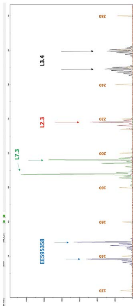
Obr. 2: Ukázka výstupu fragmentační analýzy z genetického analyzátoru pro jeden klon břízy bělokoré u čtyř mikrosatelitových markerů
