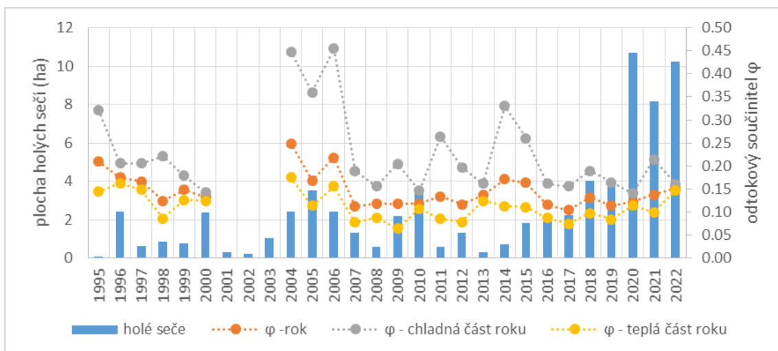
Obrázek 12: Součinitel odtoku v povodí Pekelského potoka pro období 1995–2022
