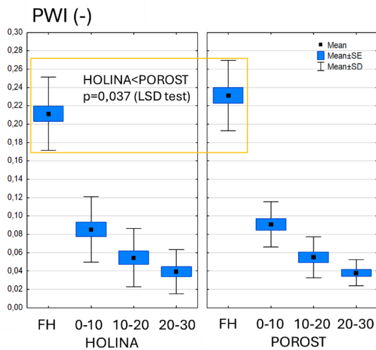
Obrázek 7: Hydrofobnost (PWI – potential wettability index) měřená v povrchovém humusu a svrchní minerální půdě na holinách a pod porostním krytem
