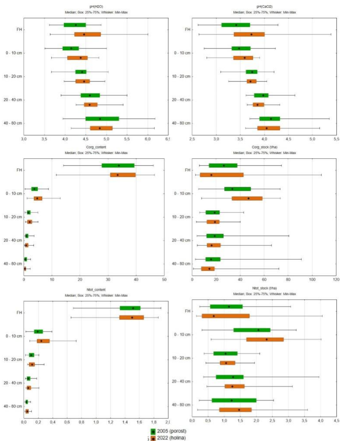
Obrázek 2: Srovnání hodnot pH, obsahu a zásoby uhlíku a dusíku v porostu a po smýcení na holině
