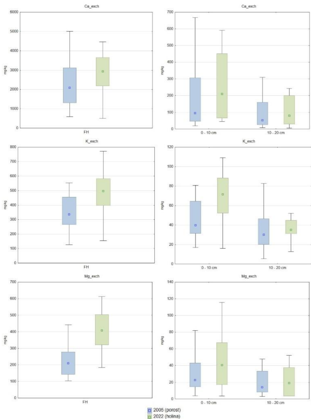
Obrázek 3: Obsah bazických živin v humusové vrstvě a ve svrchní části minerální půdy pod porostem a na holině
