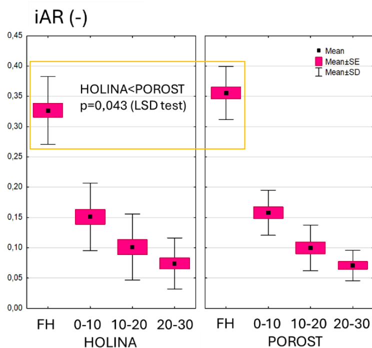
Obrázek 6: Aromaticita vyjádřená hodnotou indexu iAR ve vzorcích z holin a pod krytem porostu
