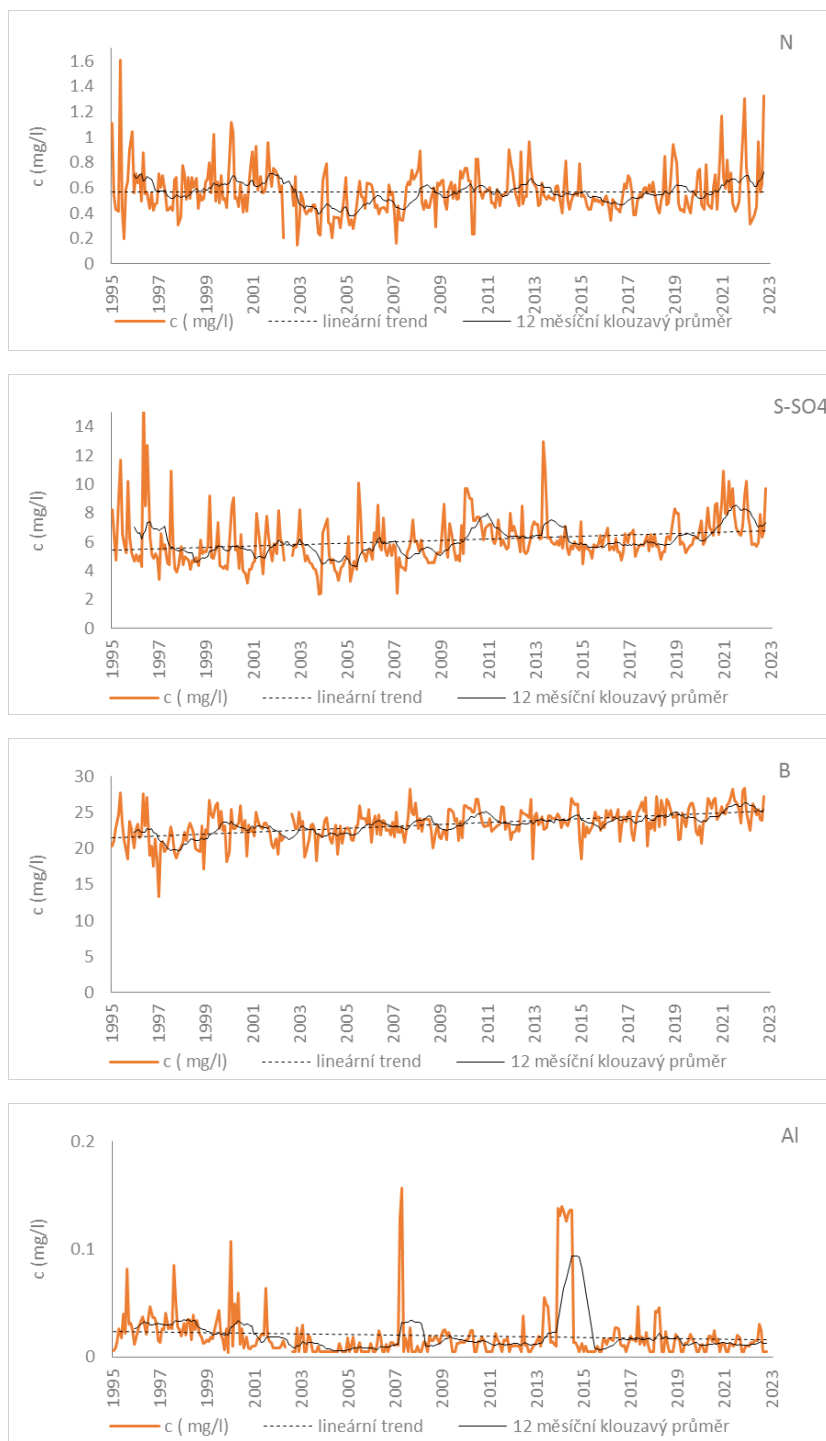
Obrázek 13: Vývoj koncentrace rozpuštěných látek ve vodě Pekelského potoka.
