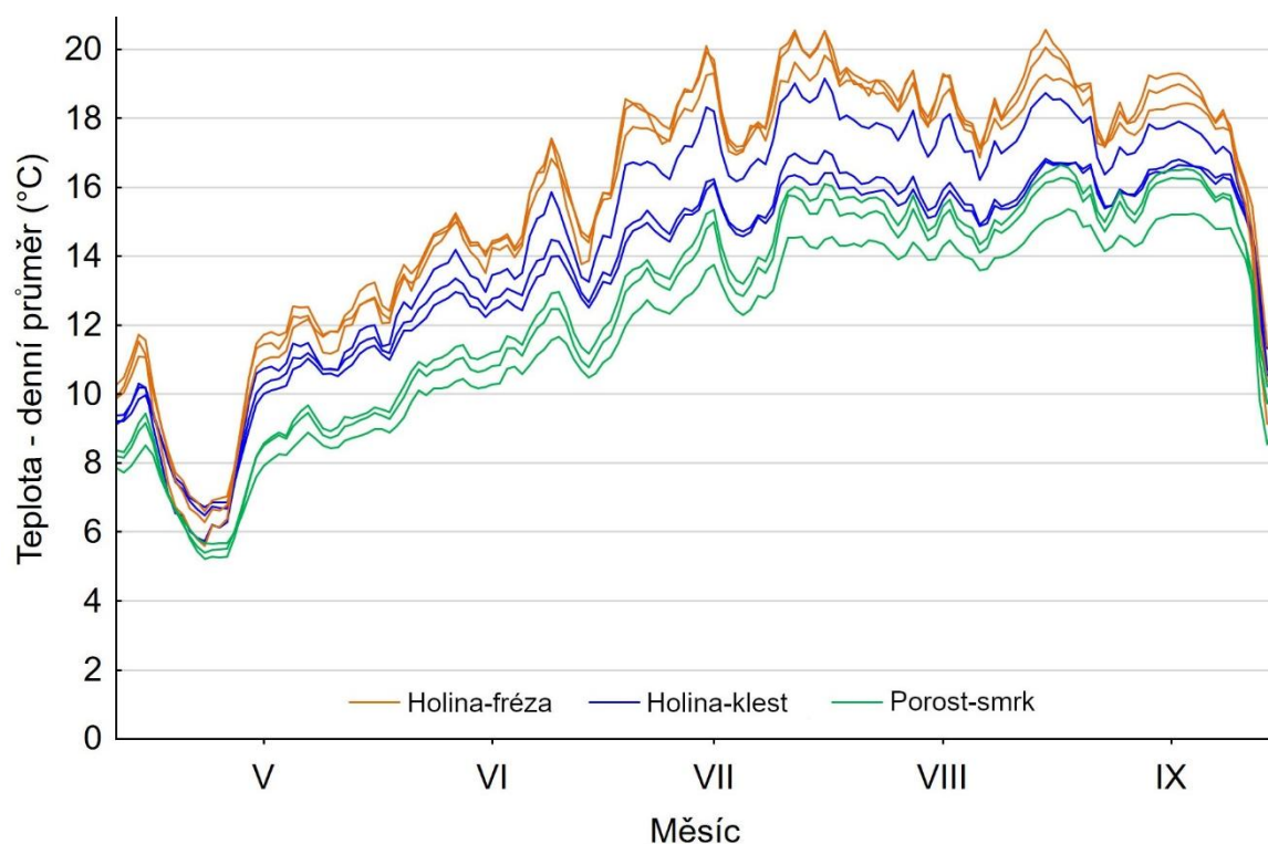
Obrázek 10: Průběhy teploty půdy v hloubce 0–10 cm na plochách kalamitních holin s frézováním povrchu vs. bez přípravy půdy a pod kontrolním porostem smrku na lokalitě Zvůle (Česká Kanada) v roce 2024.
