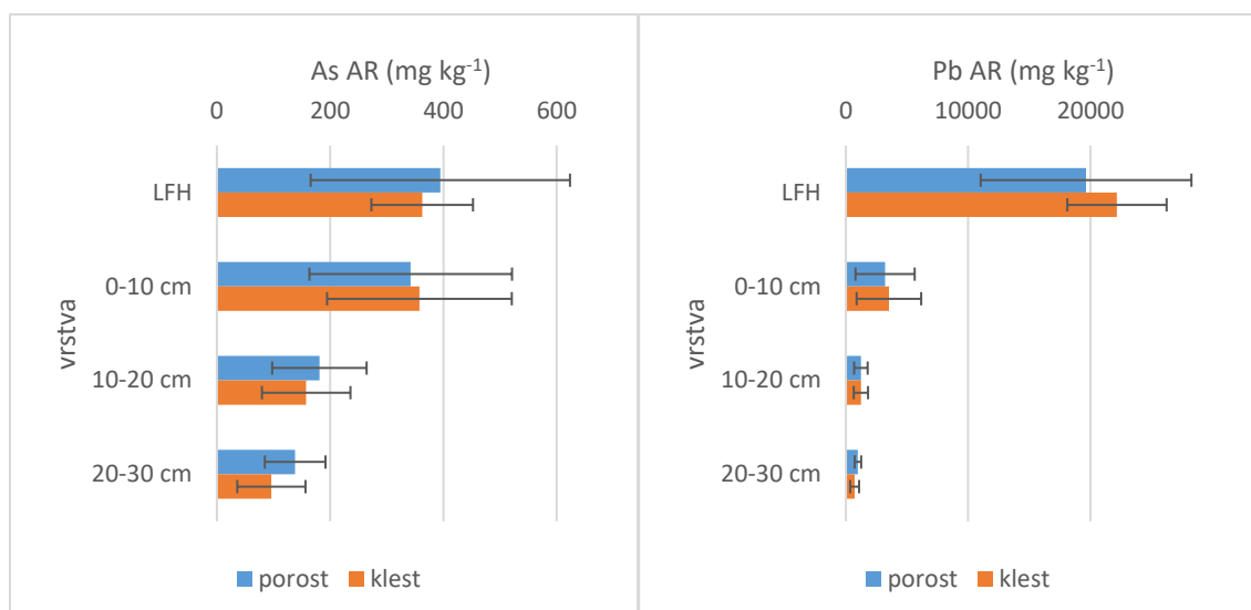
Obrázek 5. Pseudototální obsahy RP (As a Pb) extrahované lučavkou královskou (AR) v půdách pod stojícím porostem (porost) a na holinách s úklidem klestu (klest) na lokalitě Příbram (průměr a směrodatná odchylka v mg kg -1 , n = 32).
