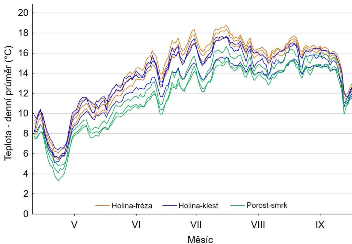
Obrazek 9: Průběhy teploty půdy v hloubce 0–10 cm na plochách kalamitních holin s drcením vs. vyklížením klestu a pod kontrolním porostem smrku na lokalitě Nové Valteřice (Hrubý Jeseník) v období V–IX 2024.
