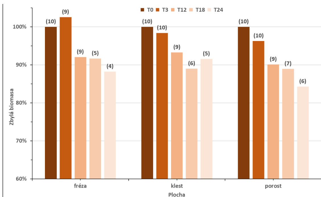
Obrázek 8: Kontingenční graf hmotnostního podílu nerozložené biomasy v průběhu dekompozice vzorků hrabanky na holých plochách s přípravou půdy frézováním, s vyklížením klestu a pod kontrolními porosty smrku v časech T 0, 3, 12, 18 a 24 měsíců od založení experimentu. Popisky sloupců udávají počty vzorků. Živé kořeny a oddenky bylinné vegetace byly ze vzorků odstraňovány od druhého odběru, podrobněji viz text.
