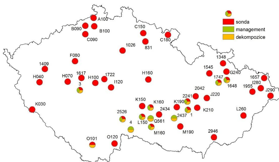
Obrázek 1: Přehled ploch zahrnutých do řešení projektu. Sonda = odběr vzorků z půdní sondy dle metodiky ICP Forests. Management = odběr vzorků ze zákopků ve variantě úklid klestu, frézování klestu a kontrola v porostu. Dekompozice = plochy se založeným dekompozičním pokusem. Podrobněji viz text.
