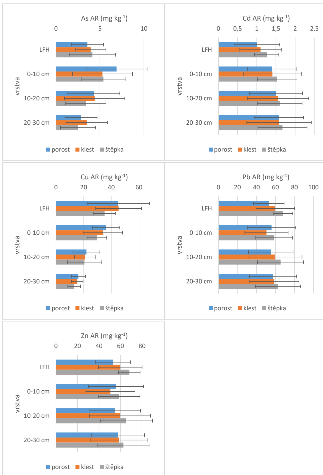
Obrázek 4: Pseudototální obsahy RP (As, Cd, Cu, Pb, Zn) extrahované lučavkou královskou (AR) v půdách pod stojícím porostem (porost) a na holinách s úklidem klestu (klest) a drcením klestu (štěpka) (průměr a směrodatná odchylka v mg kg -1 , n = 145). Jedná se o průměry z lokalit s běžnými hodnotami rizikových prvků.
