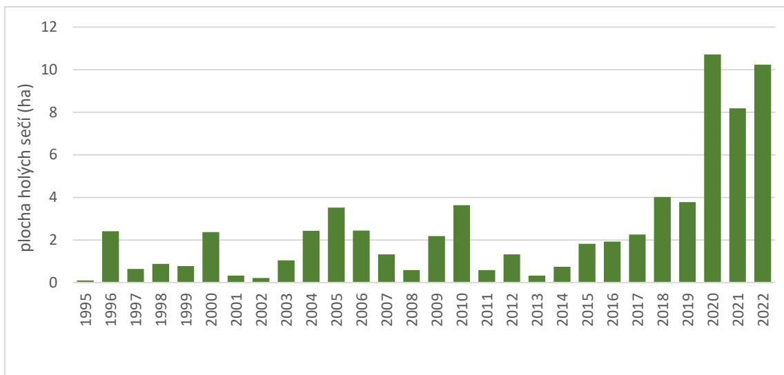
Obrázek 11: Plochy holých sečí v povodí Pekelského potoka detekované z multispektrálních snímků družice Landsat.
